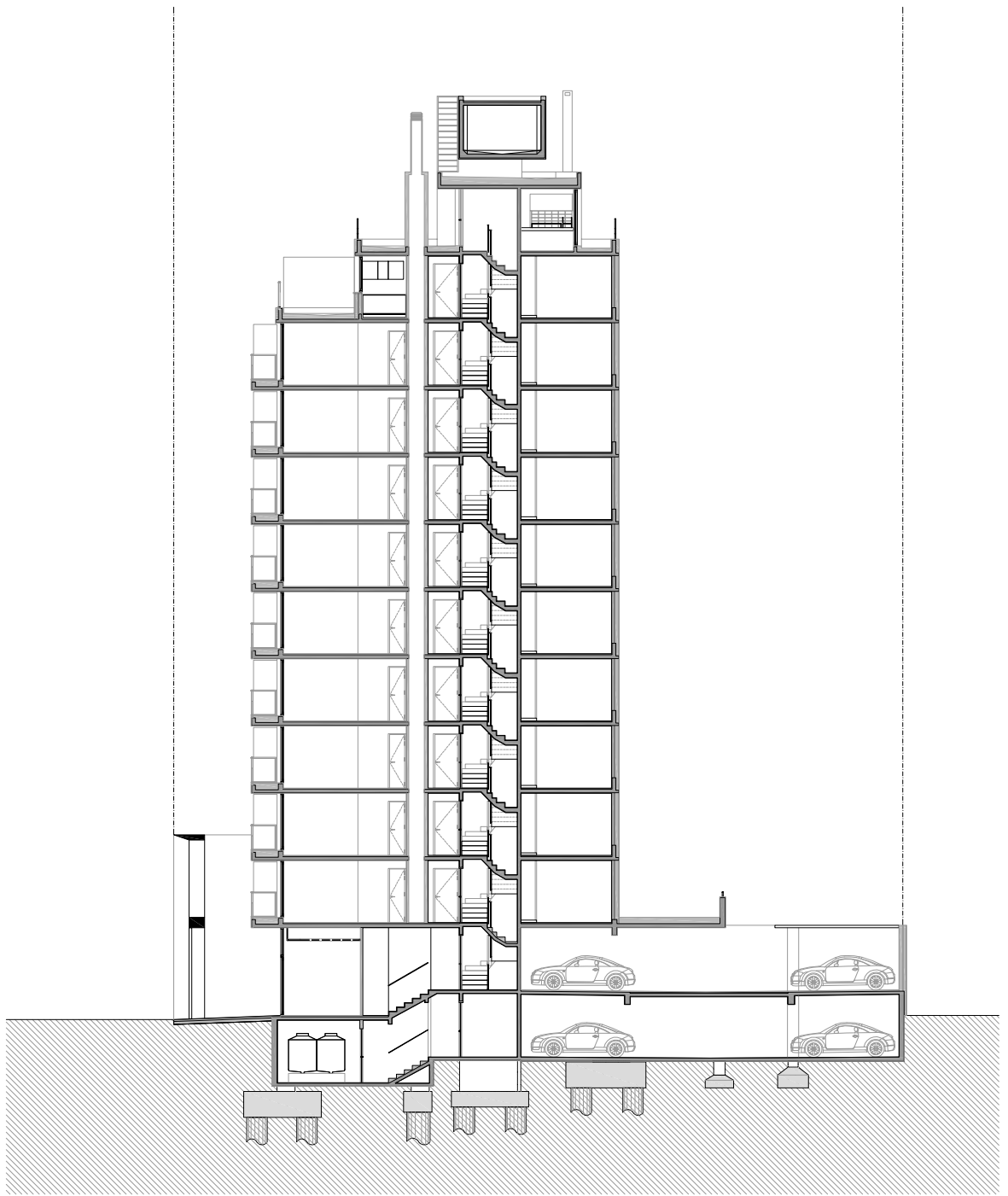
CORTE AA
